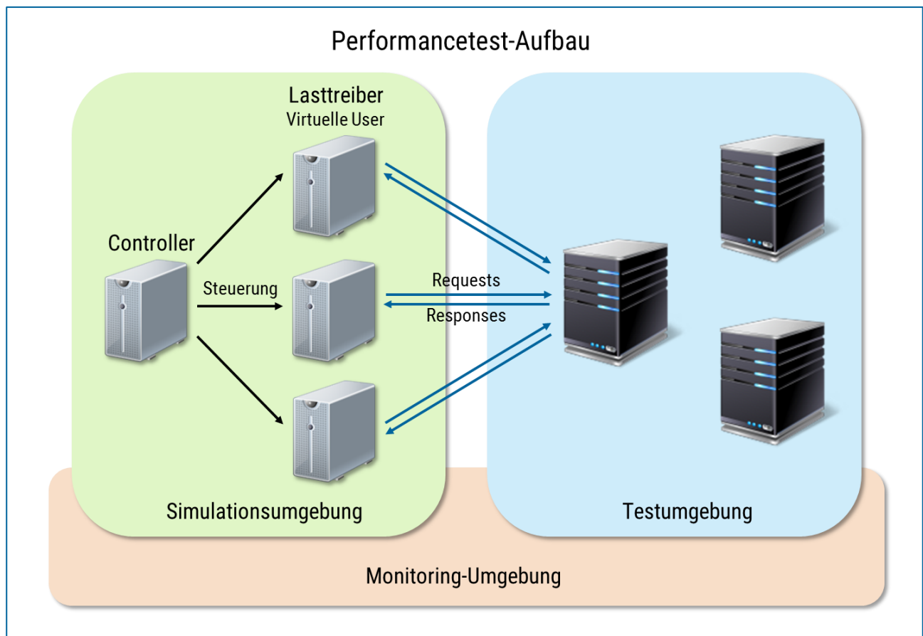
Abbildung 1: Experimenteller Aufbau eines Performancetests. Die Lasttreiber, die durch den Controller gesteuert werden, simulieren virtuelle User. Diese führen skriptbasiert bestimmte Folgen von Requests gegen das zu testende System aus. Unterdessen werden die zugehörigen Request-Response-Zeiten von den virtuellen Usern und anderweitige Systemreaktionen durch entsprechende Monitore gemessen.
