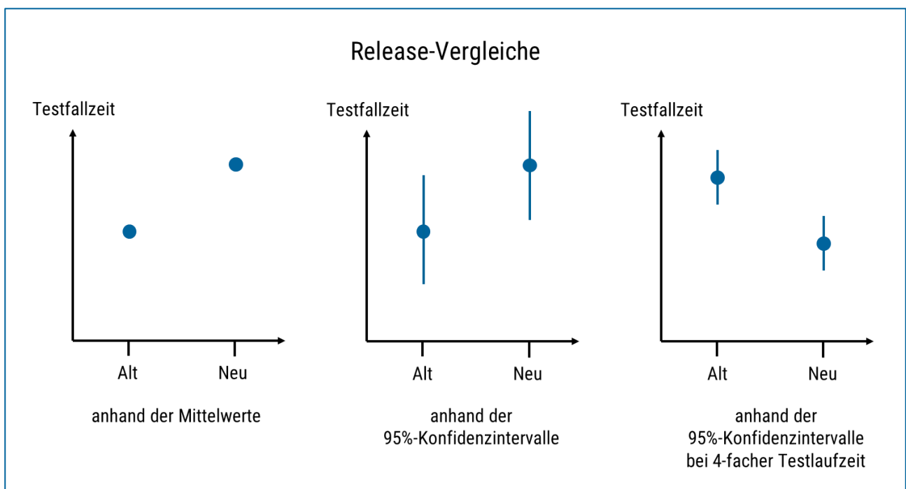
Abbildung 3: Man stelle sich vor, dass mehrere gleichartige Performancetests mit konstanter virtueller Userzahl und einem einzigen Testfall gegen Release Alt und Release Neu durchgeführt wurden, um die damit verbundenen Performance-Unterschiede zu bestimmen. Links: Der Vergleich der Mittelwerte der Testfallzeiten ist wertlos, weil daraus nicht erkennbar ist, wo die Mittelwerte bei erneuter Durchführung der Tests lägen. Mitte: Bei Hinzunahme der 95%-Konfidenzintervalle sehen wir, dass die Tests etwaige Performance-Unterschiede nicht auflösen können, weil sich die Intervalle in beträchtlicher Weise überdecken. Rechts: Bei erneuter Durchführung der Tests mit vierfacher Testlaufzeit halbieren sich die Konfidenzintervalle. Diese liegen nun überschneidungsfrei auseinander, so dass ein signifikanter Performance-Unterschied konstatiert werden kann.
